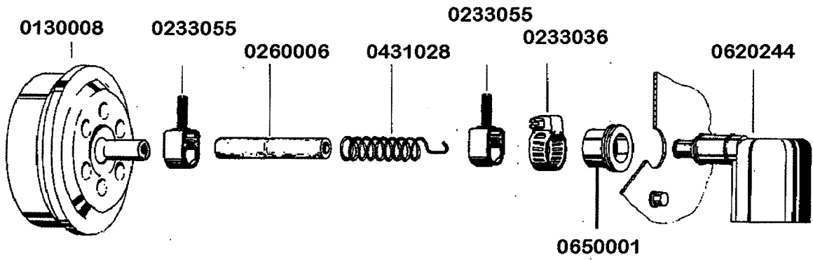
0130001 Niveauschalter MK2 - Platine
